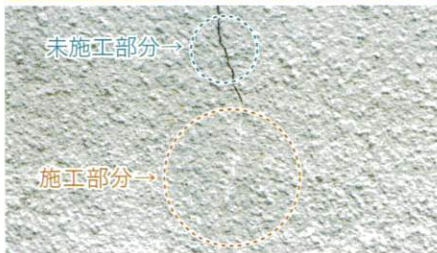
■施工終了後 HSS工法施工状況の比較
